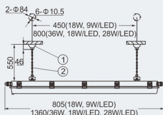
D: pendant chain type
