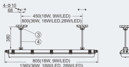
G: pendant pole type
