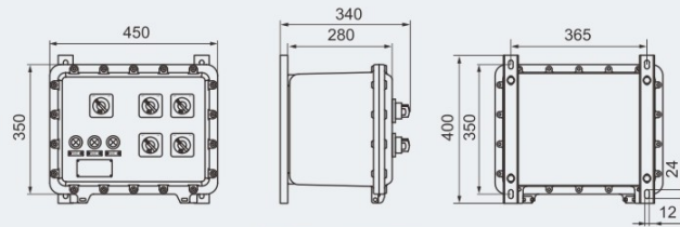
BXM81-4/□/□/□
