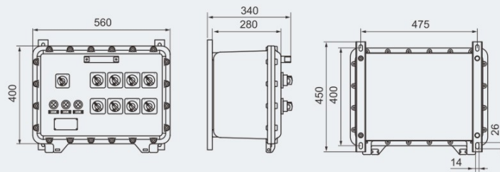
BXM81-8/□/□/□
