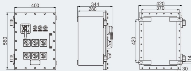
BXM(D)81-6/□/□/□
