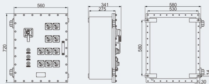
BXM(D)81-10/□/□/□
