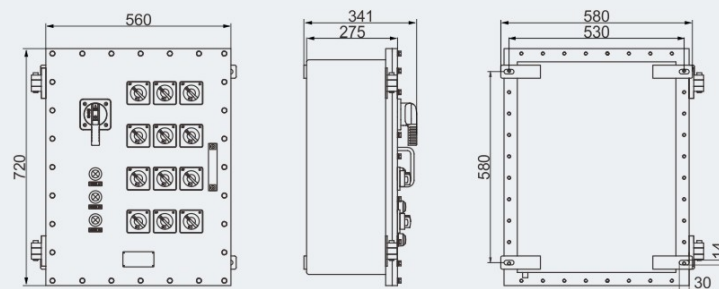
BXM(D)81-12/□/□/□
