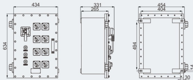
BXM(D)81-8/□/□/□
