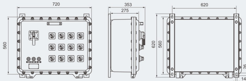
BXM81-12/□/□/□
